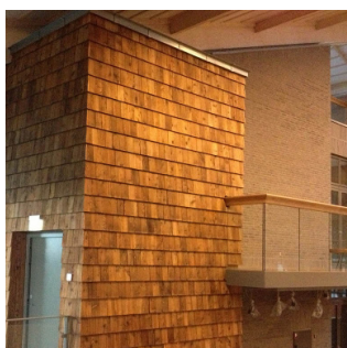
Forpatineret og brandimpregneret Lærk efterbehandlet med TD-olie.
